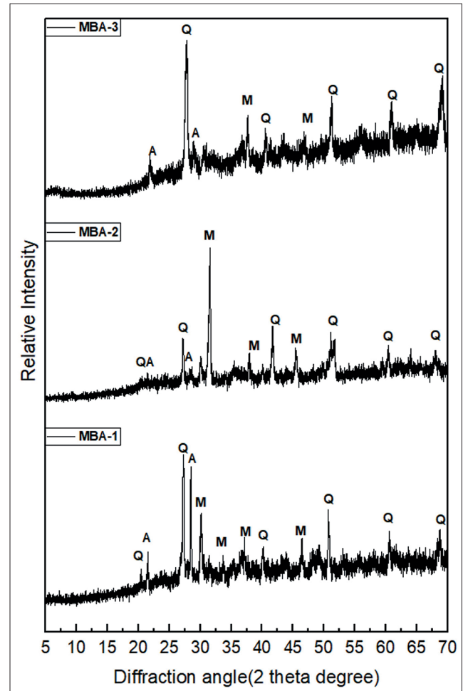
Figure 10. XRD results of MBA mud brick samples. (Q: Quartz, A: Anorthite, M: Muscovite)/MBA kerpiç buluntularının XRD sonuçları. (Q: Kuvars, A: Anortit, M: Muskovit).
