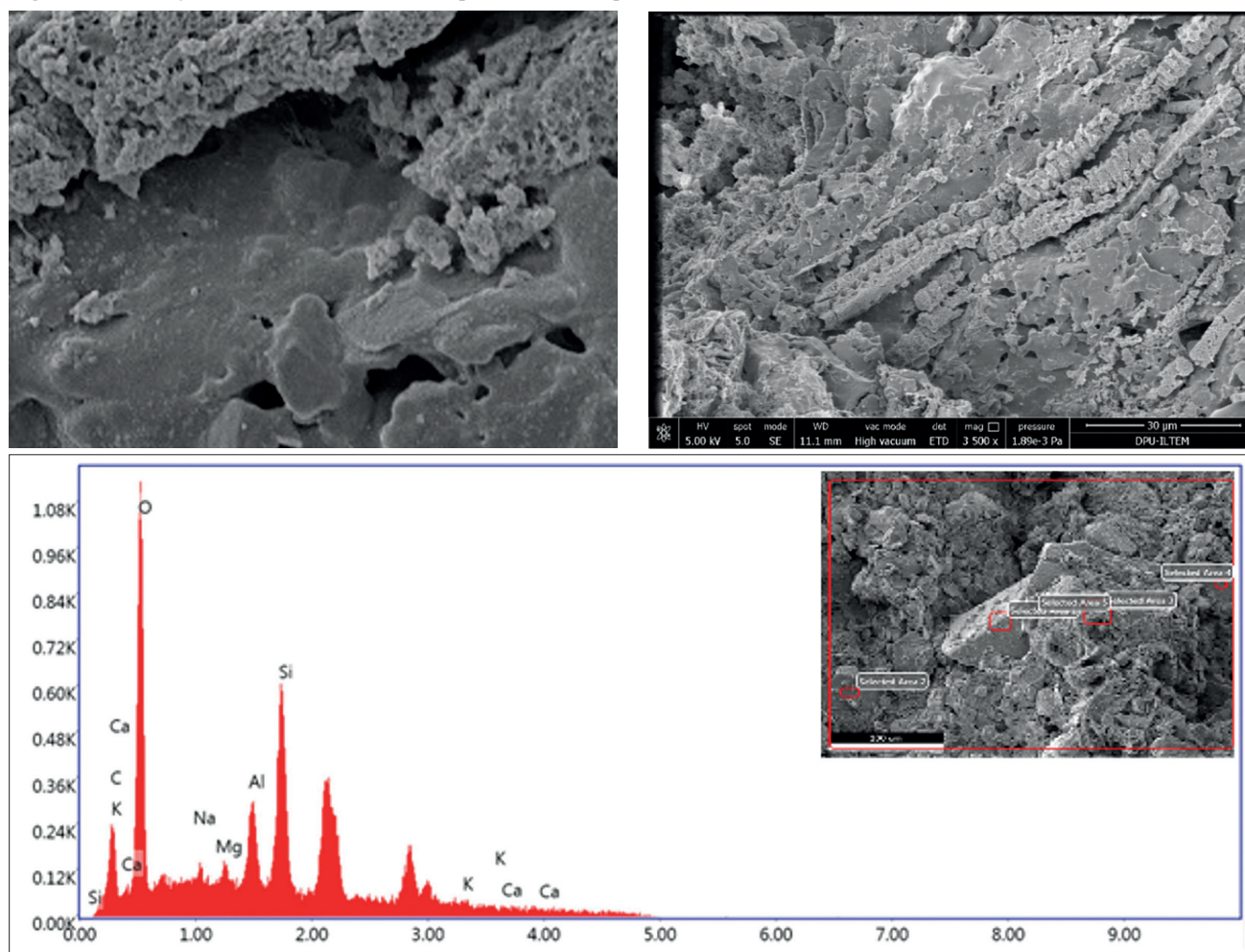
Fig. 17. SEM analysis of MBA-3 mud brick samples / MBA-3 kerpiç buluntularının SEM analizi.
